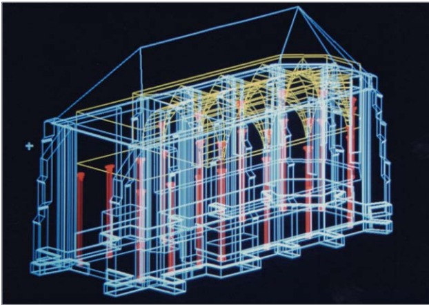
Abb. 88: Forschungsprojekt M. Schwarz: Versuch der Positionierung der Gewölbe der Capella Speciosa am ersten Drahtgittermodell. Axonometrische Darstellung. (Michael Mayr-Ebert).
