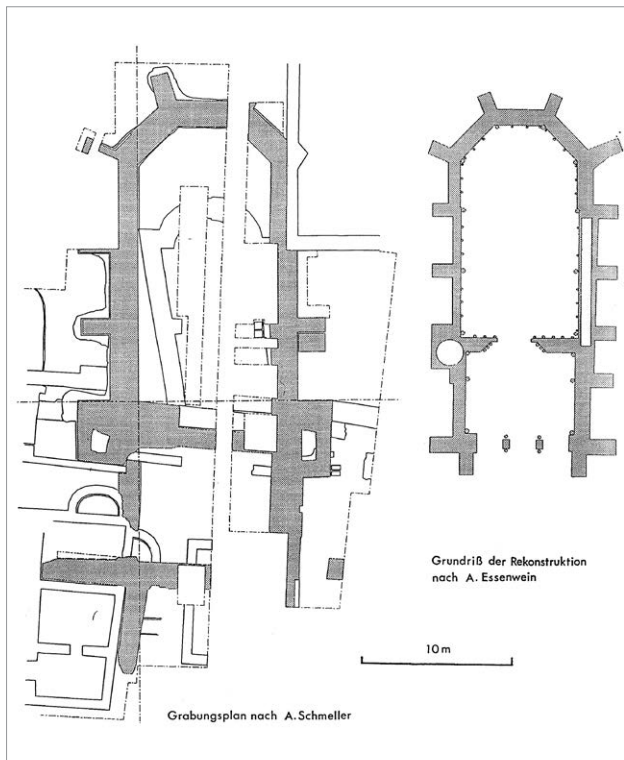
Abb. 84: Forschungsprojekt M. Schwarz: Maßstäblicher Vergleich des von A. Schmeller publizierten Grabungsplanes mit dem Grundriß der Rekonstruktion von A. Essenwein. (Mario Schwarz).
