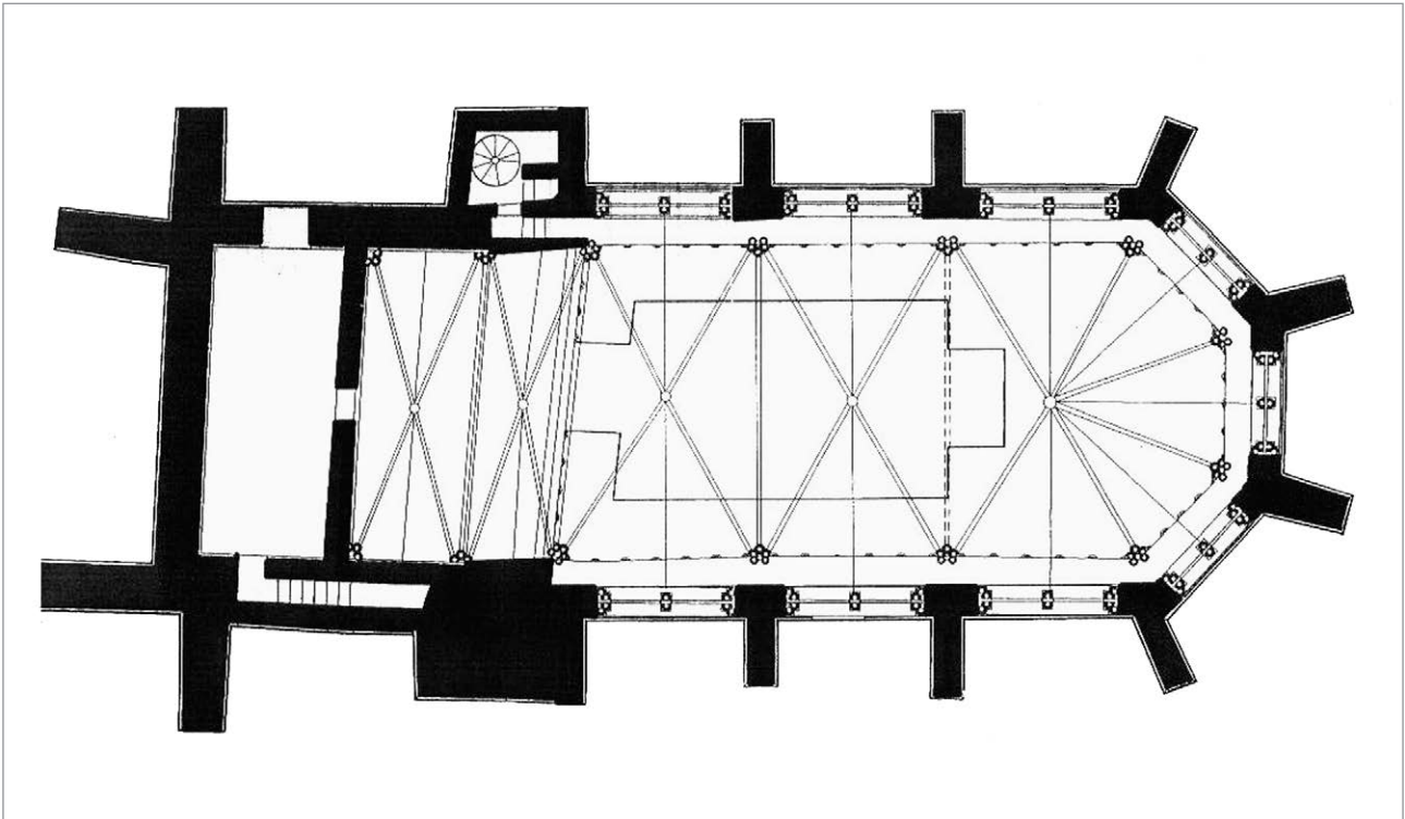
Abb. 92: Forschungsprojekt M. Schwarz: Grundriss der Rekonstruktion der Capella Speciosa. (Elmar Schmidinger).
