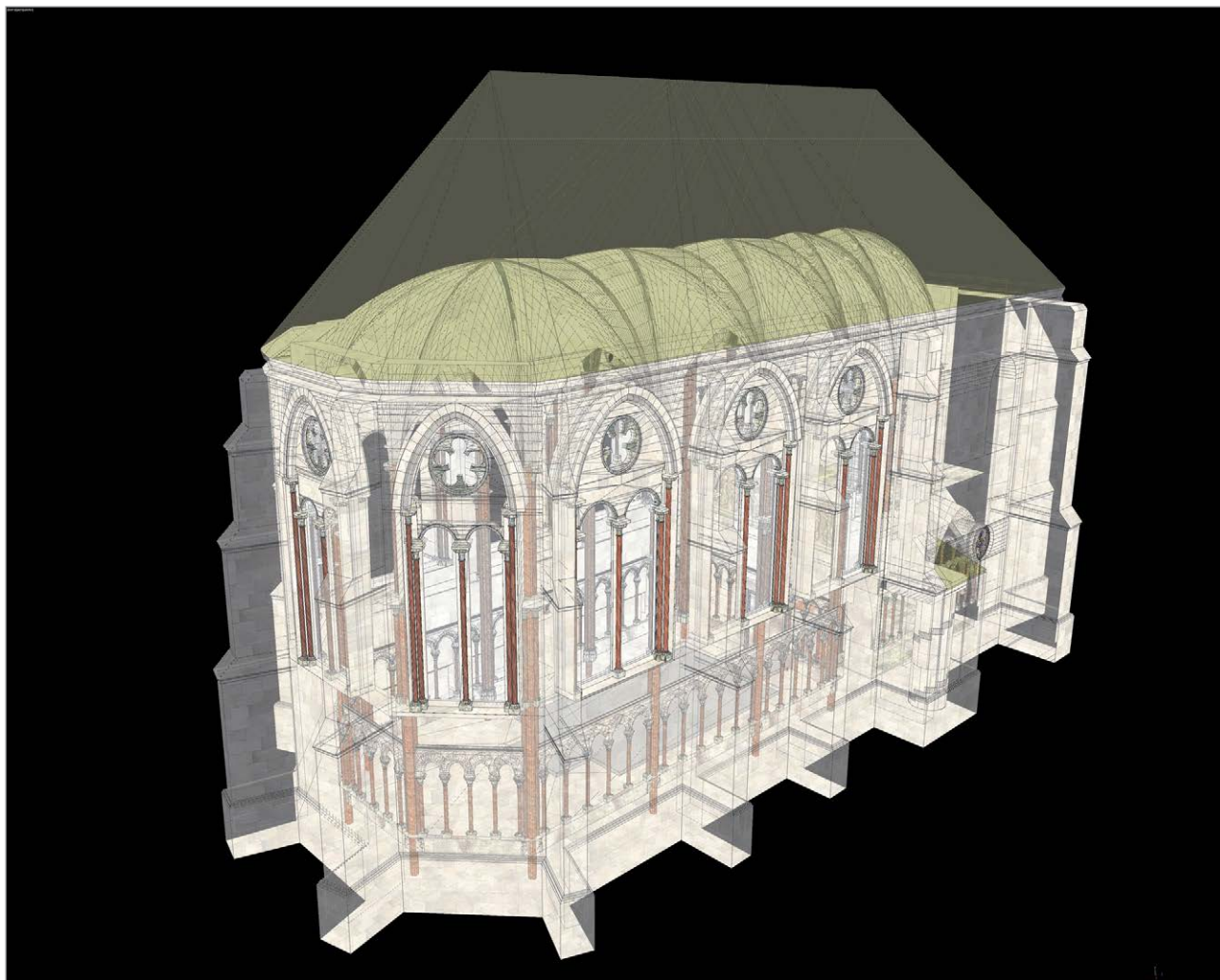
Abb. 99: Forschungsprojekt M. Schwarz: Semitransparente perspektivische Visualisierung der Rekonstruktion der Capella Speciosa. Ansicht von Nordosten. (Elmar Schmidinger).
