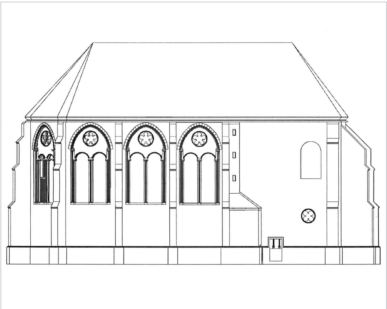
Abb. 93: Forschungsprojekt M. Schwarz: Aufrissansicht der Nordseite der Rekonstruktion der Capella Speciosa. (Elmar Schmidinger).
