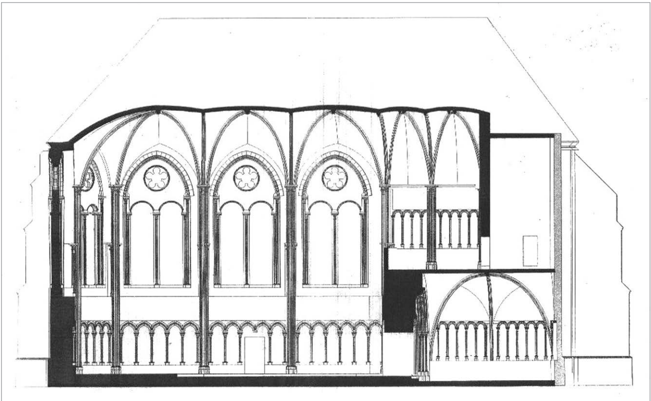
Abb. 94: Forschungsprojekt M. Schwarz: Aufrisschnitt der Rekonstruktion der Capella Speciosa. Schnittebene in der Längsachse, Blick nach Süden. (Elmar Schmidinger).
