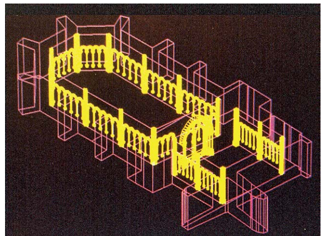
Abb. 87: Forschungsprojekt M. Schwarz: Versuch der Positionierung der Gewölbeträger, der Blendarkaden und des Westportals der Capella Speciosa am ersten Drahtgittermodell. Axonometrische Darstellung. (Michael Mayr-Ebert).
