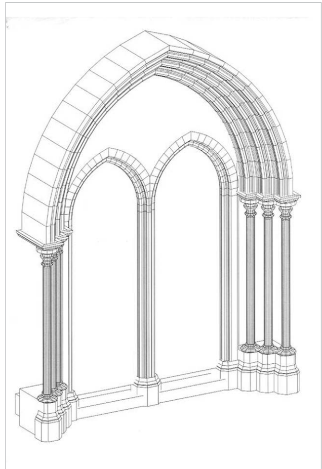
Abb. 85: Forschungsprojekt M. Schwarz: Versuch der digitalen Erfassung des Portals aus der Capella Speciosa. Axonometrische Darstellung. (Michael Mayr-Ebert).
