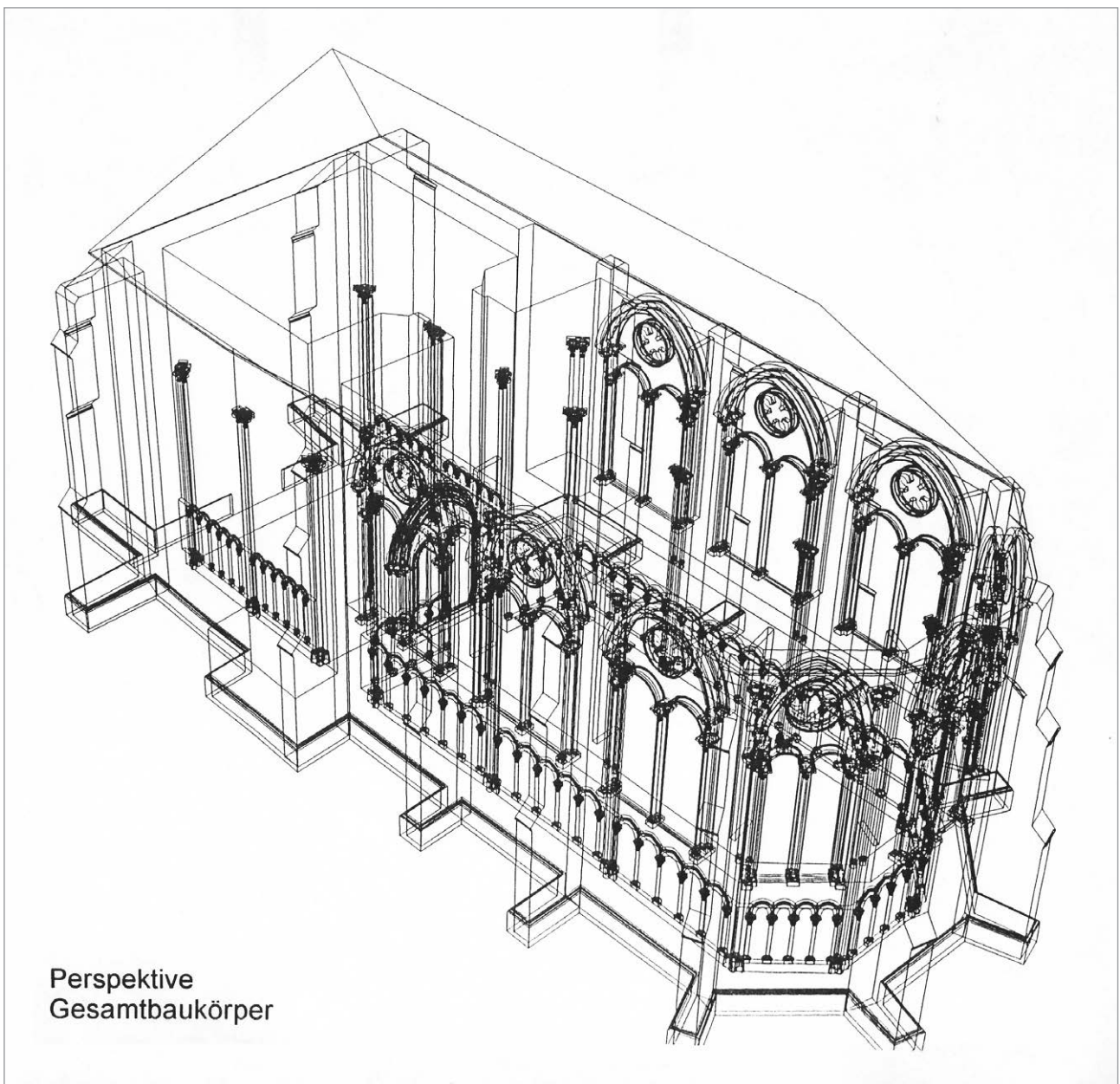
Abb. 89: Forschungsprojekt M. Schwarz: Positionierung der Fenster der Capella Speciosa am überarbeiteten Drahtgittermodell. Axonometrische Darstellung. (Elmar Schmidinger).
