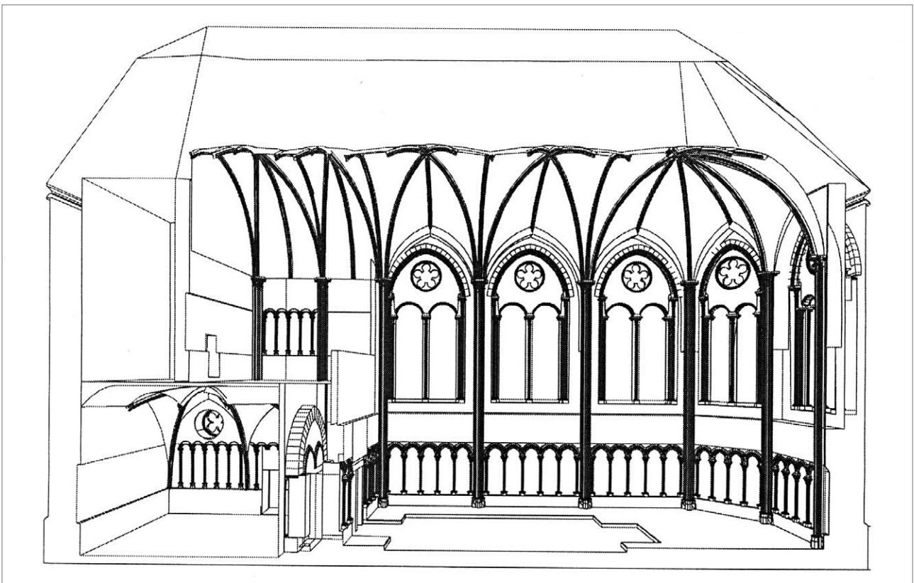
Abb. 98: Forschungsprojekt M. Schwarz: Rekonstruktion der Gewölbe und der Westempore der Capella Speciosa in aufgeschnittener Perspektive. Schnittebene parallel zur Längsachse. Gerenderter Strichzeichnung. (Elmar Schmidinger).
