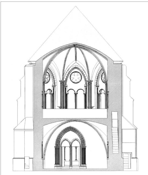
Abb. 95: Forschungsprojekt M. Schwarz: Aufrisschnitt der Rekonstruktion der Capella Speciosa. Schnittrichtung im rechten Winkel zur Längsachse, Schnittebene durch Vorhalle und Westempore. Blick nach Osten. (Elmar Schmidinger).
