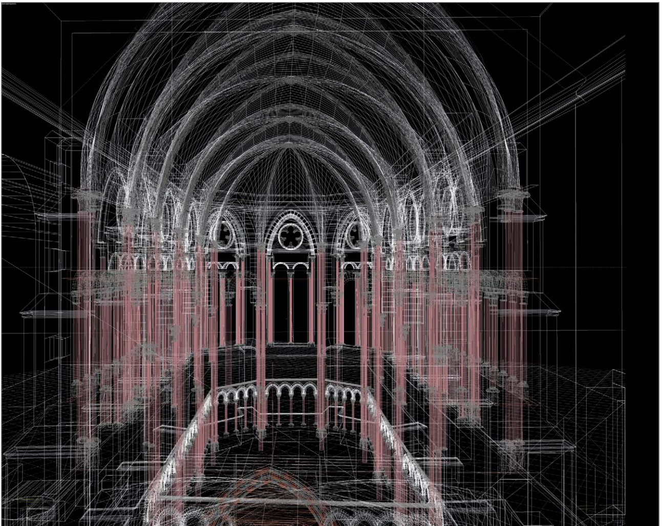
Abb. 91: Forschungsprojekt M. Schwarz: Konstruktion der Gewölbe der Capella Speciosa am überarbeiteten Drahtgittermodell. Perspektivische Darstellung mit Blick nach Osten. (Elmar Schmidinger).
