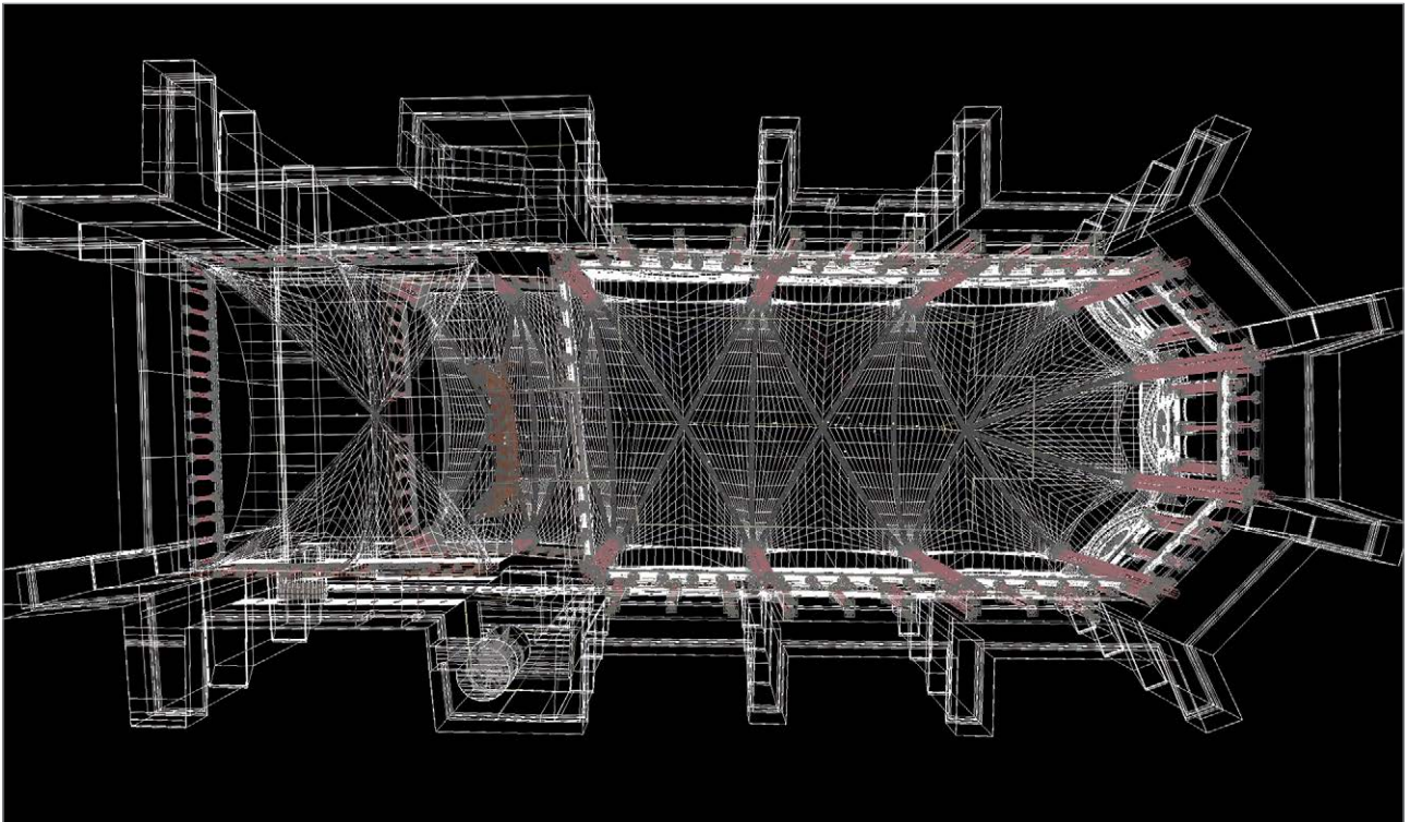
Abb. 90: Forschungsprojekt M. Schwarz: Konstruktion der Gewölbe der Capella Speciosa am überarbeiteten Drahtgittermodell. Perspektivische Darstellung in Untersicht. (Elmar Schmidinger).
