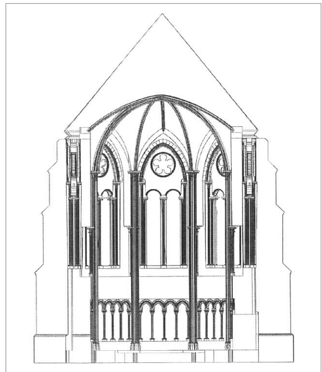
Abb. 96: Forschungsprojekt M. Schwarz: Aufrisschnitt der Rekonstruktion der Capella Speciosa. Schnittrichtung im rechten Winkel zur Längsachse, Schnittebene durch das Presbyterium. Blick nach Osten. (Elmar Schmidinger).
